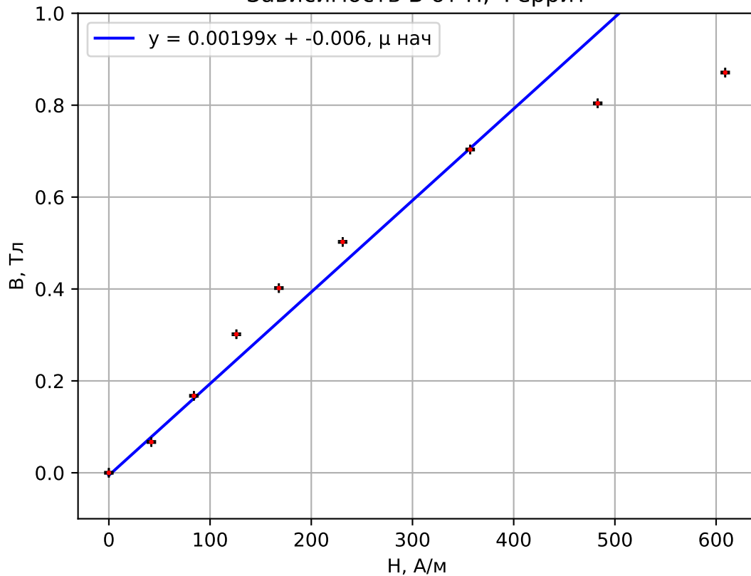
Зависимость В от Н, Феррит
